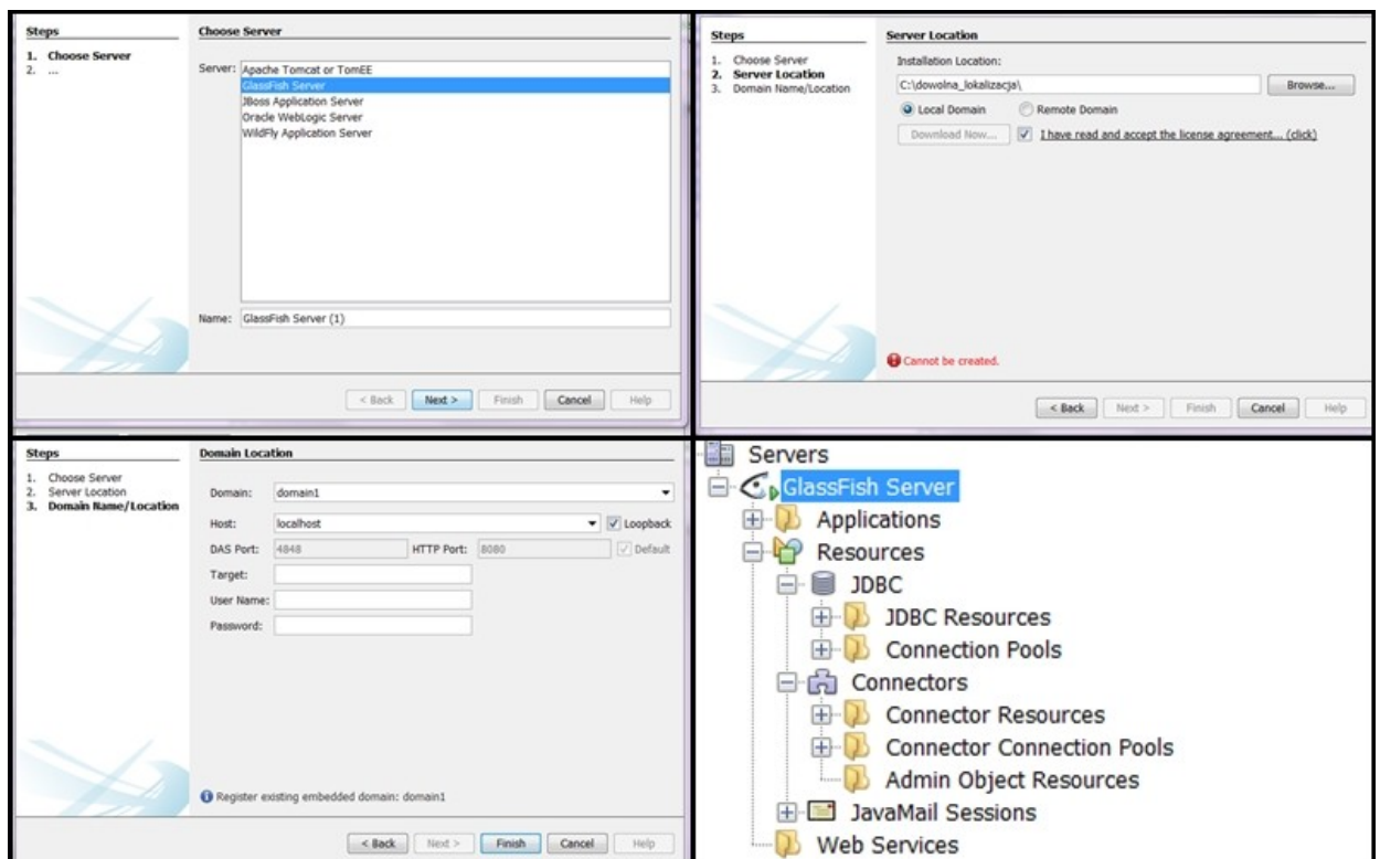
Rys. 2: Zrzuty ekranu / środowisko NetBeans 8.02 (okna wstępnej konfiguracji połączenia z serwerem; widok zawartości GlassFish z poziomu IDE)
